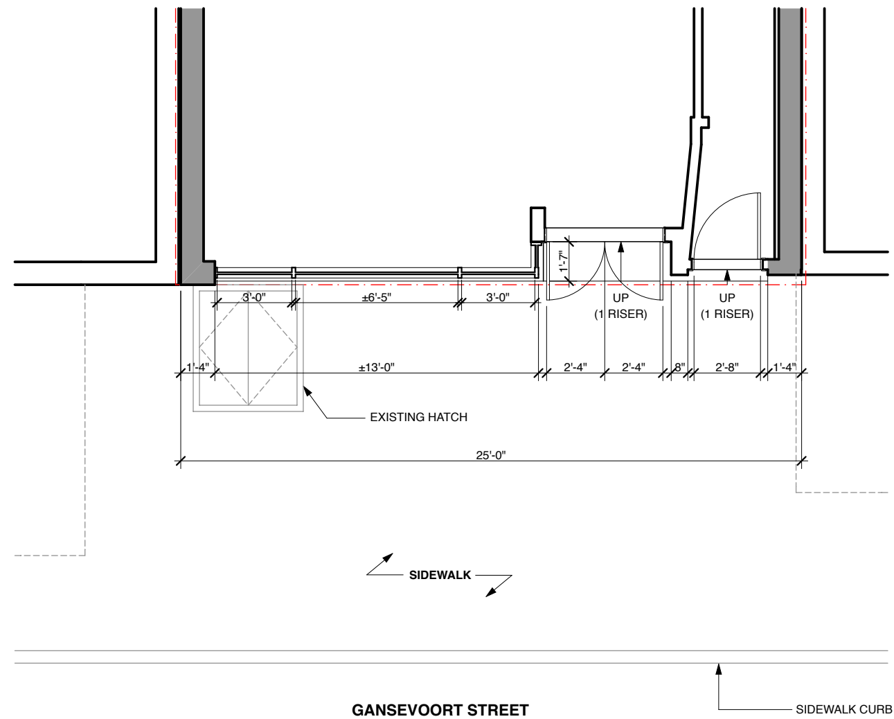
1 EXISTING STOREFRONT PLAN SCALE: 3/16" = 1'-0"
